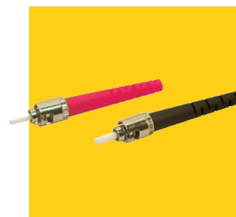
Konektor ST
